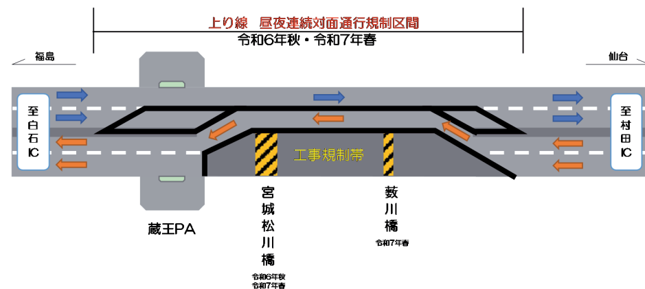
図 1: 昼夜連続対面通行規制区間 概要図
