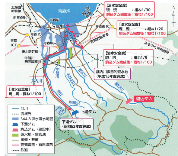
図・2 駒込ダムの治水効果概要
