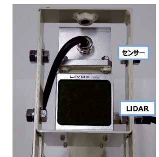
センサーユニット写真
