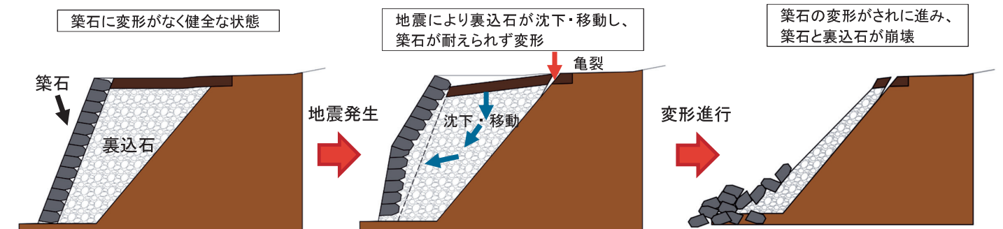
図-5 崩落順序
