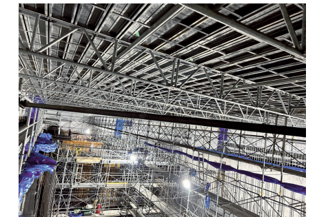
〔写真-4〕雪寒仮囲い
